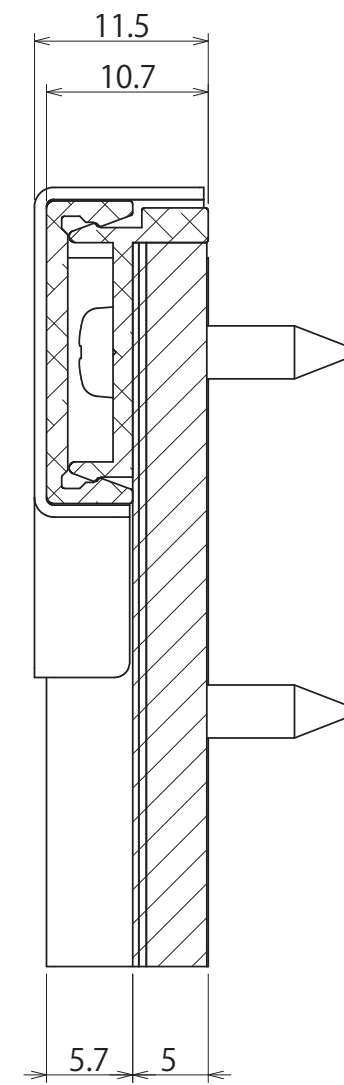
断面図 A-A スケール 2:1
